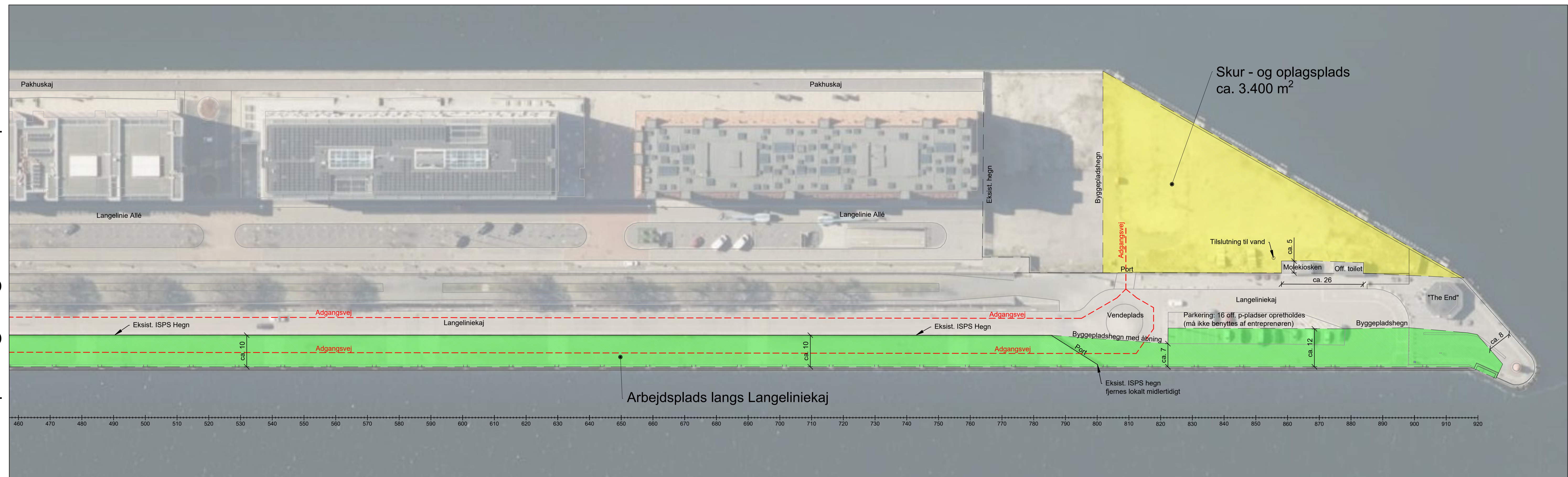
Byggeplan af Langelinie kaj, 1:700
